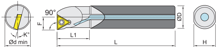
Coolant carbide shank (Right-hand shown) 中心出水鎢鋼柄 右向示意圖
