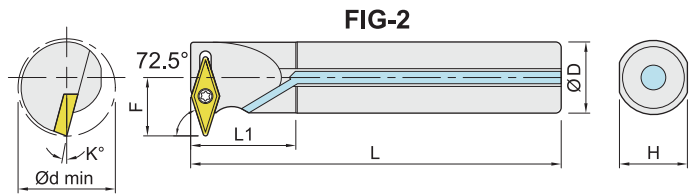
FIG-2 Coolant steel shank (right shown) 中心出水鋼柄 右向示意圖
