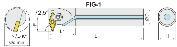
FIG-1 Coolant steel shank+clamp (right shown) 中心出水鋼柄+壓板 右向示意圖
